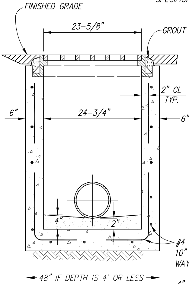
SECTION A-A
